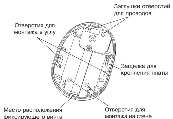
Рисунок 3 – Основание извещателя
